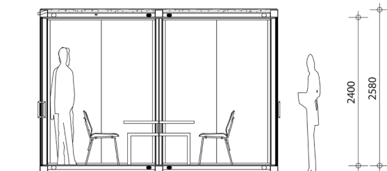
DOORSNEDE
