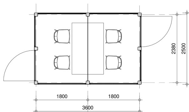
PLATTEGROND ALS PALAVERBOX
