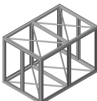
CONSTRUCTIE
