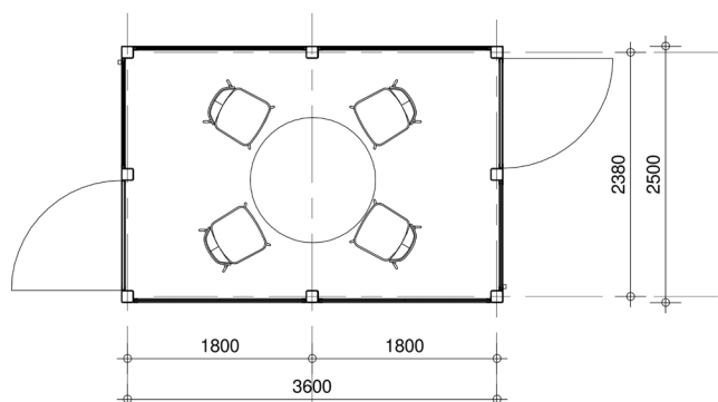
PLATTEGROND ALS THEEHUISJE
